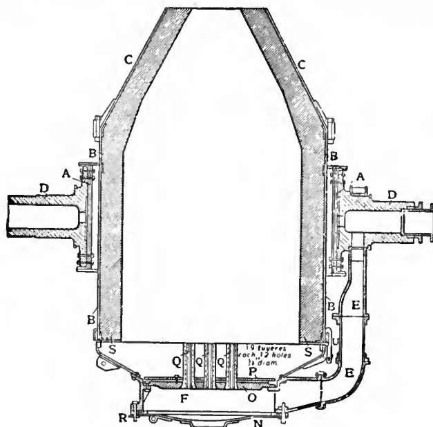
FIG. 16.—12-15 ton Bessemer Converter.
